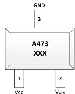
SOT23-3L
