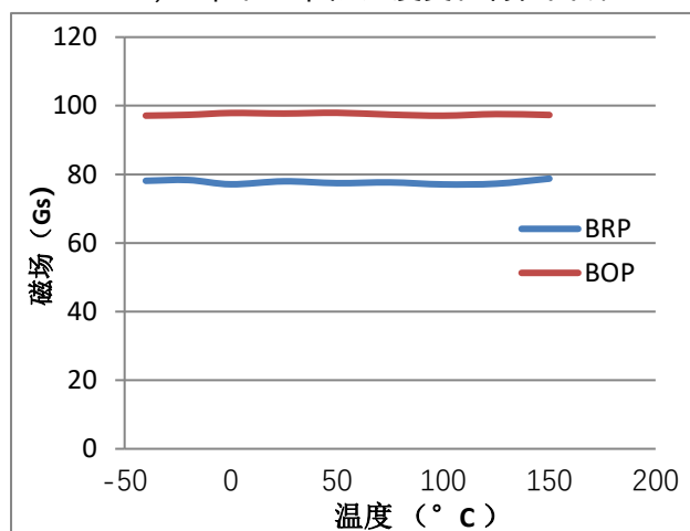
V_{CC}=5V , Bop 和 Brp 随温度变化特性曲线
