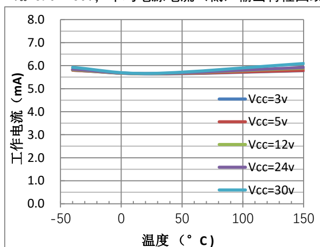
V_{CC}=3.0\sim30V , 平均电源电流（低）输出特性曲线
