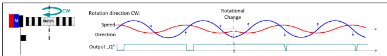
设置 “EDGE_POLAR = 0” 和 “FORWARD_DEF” = 1 时的信号输出
