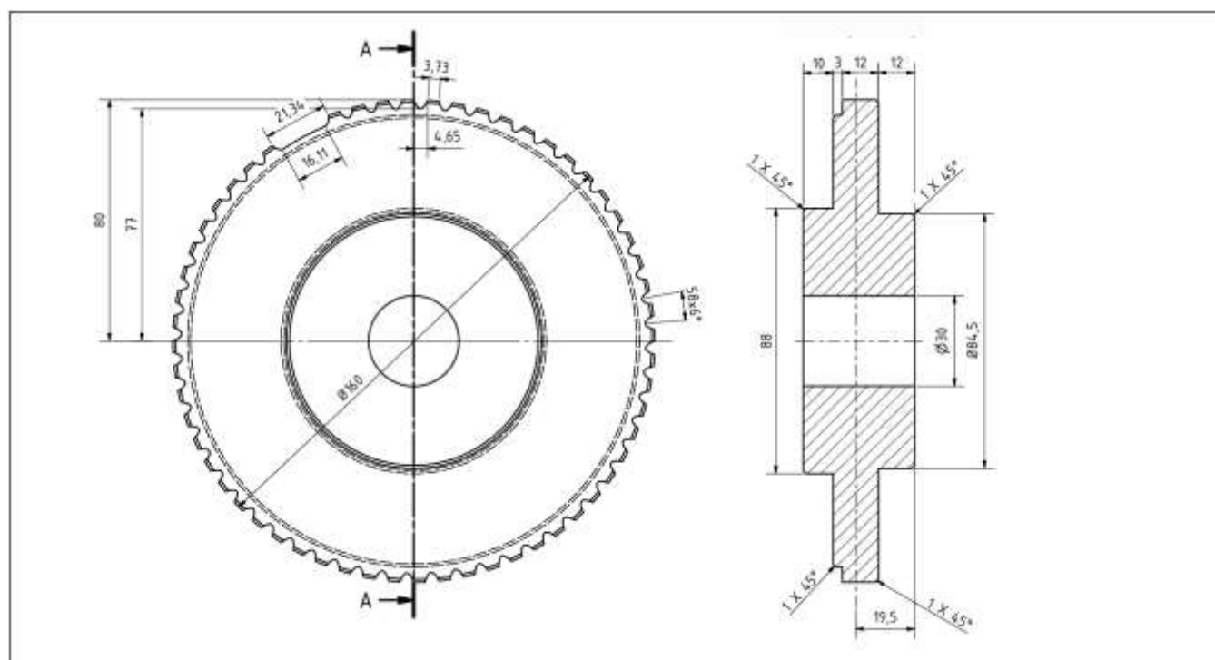
OEM-曲轴轮（外径 = 160mm）
