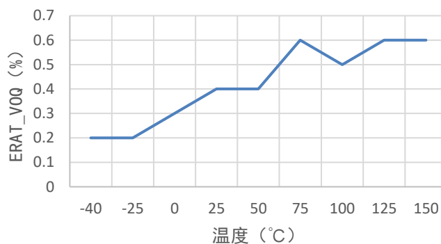
静态输出误差随温度变化
