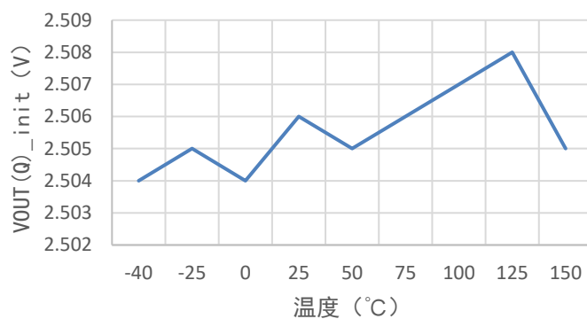
0A电流，输出随温度变化
